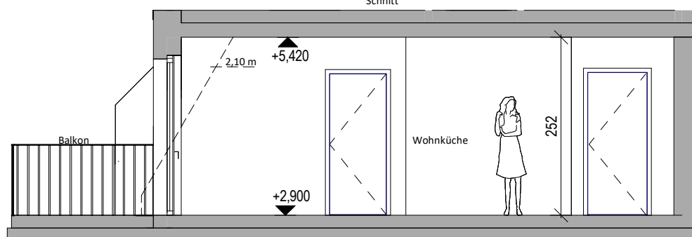
Schnitt 1:75
