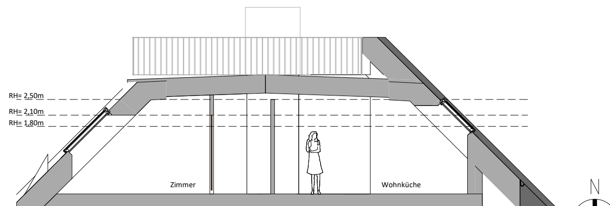
SCHNITT 2
