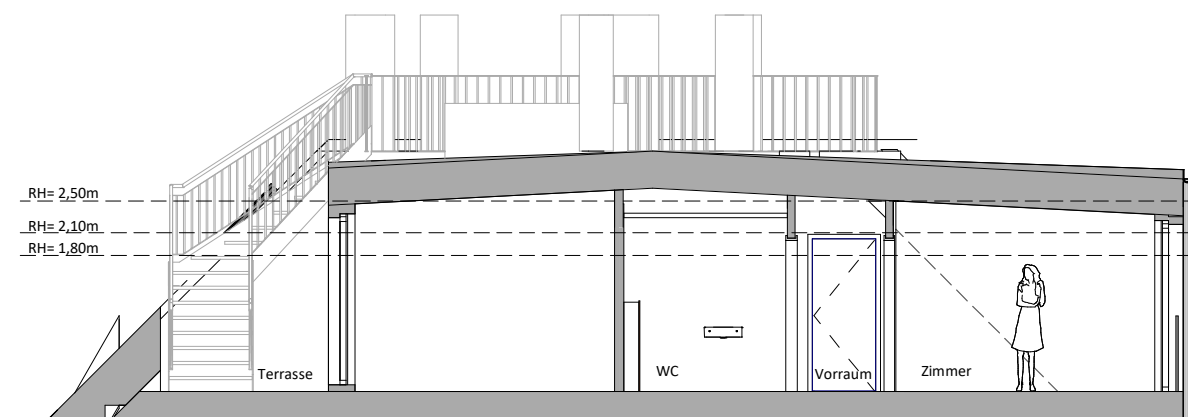
SCHNITT 2
