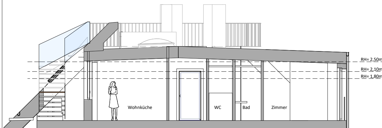
SCHNITT 1
