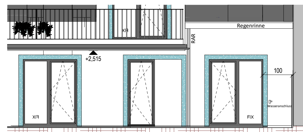
Hofansicht
