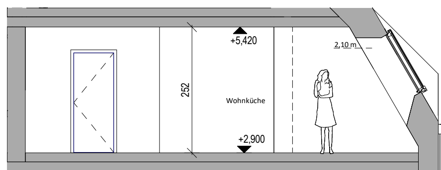
Schnitt 1:75
