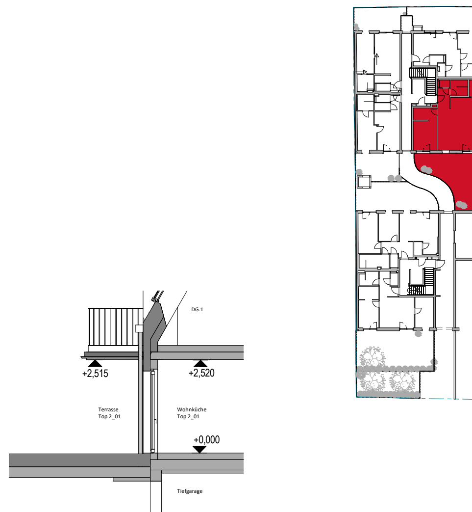
Schnitt
