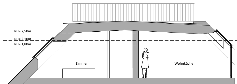
SCHNITT 1
