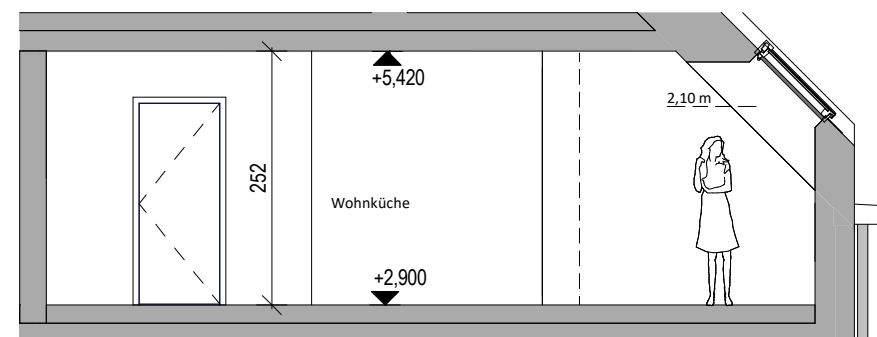
Schnitt 1:75
