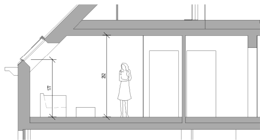
SCHNITT
